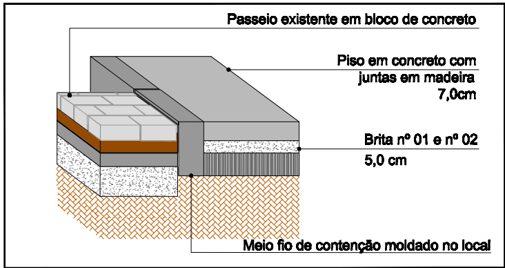
02 | CORTE ESQUEMÁTICO - ENCONTRO DE PAVIMENTOS
