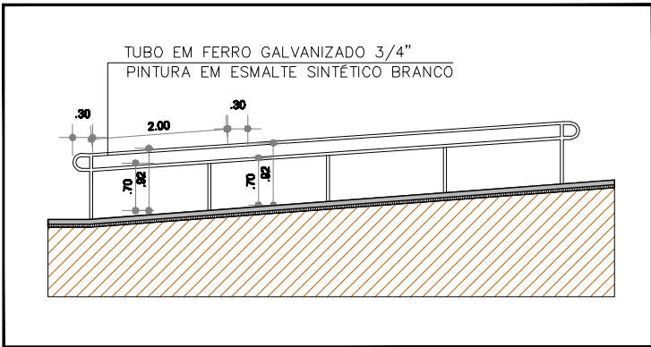
03 | DETALHAMENTO CORRIMÃO ACESSO PRINCIPAL
