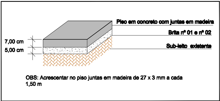
04 | CORTE ESQUEMÁTICO - PISO CIMENTADO - PASSEIO
